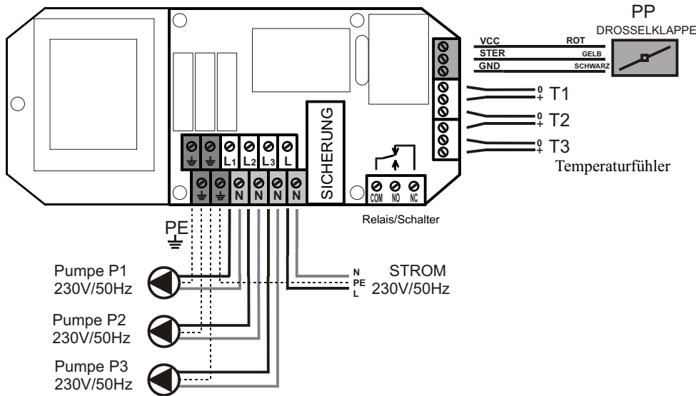
Abb. 3 Elektroinstallationschema
